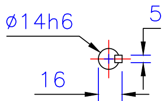
输入轴 Input shaft
